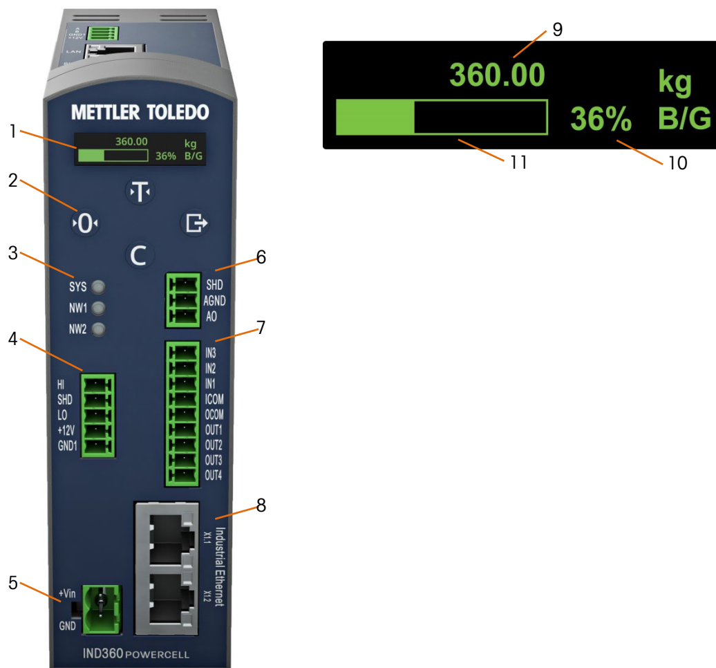
图 1-1: 智能料罐称重应用程序界面-IND360DIN 导轨式
