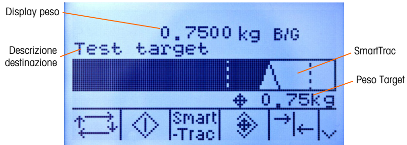
Figura 2-14: SmartTrac Trasferimento materiali di media dimensione
