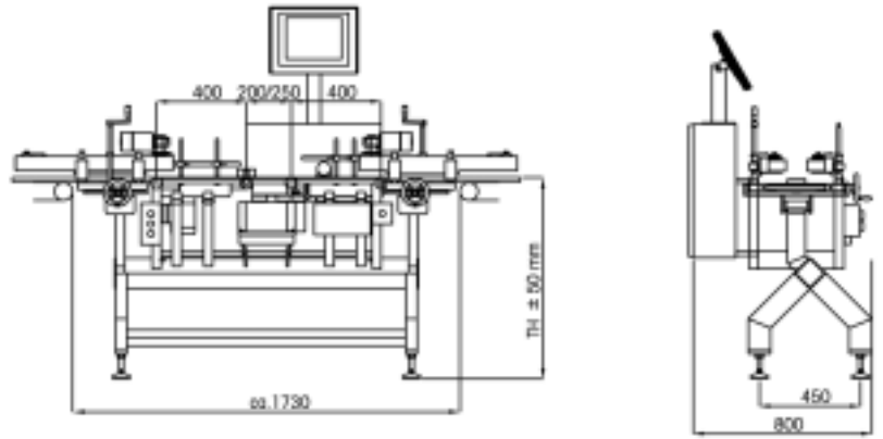
链式自动检重秤(在输入/输出安装产品侧面夹持传输装置)
